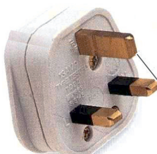
earthing • la mise à la terre die Erdung • la toma de tierra la messa a terra • ligação à terra
